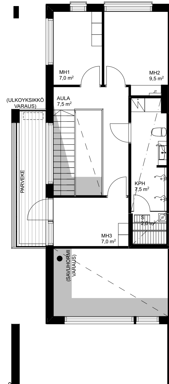
POHJAPIIRROS 2.KRS 1:100
