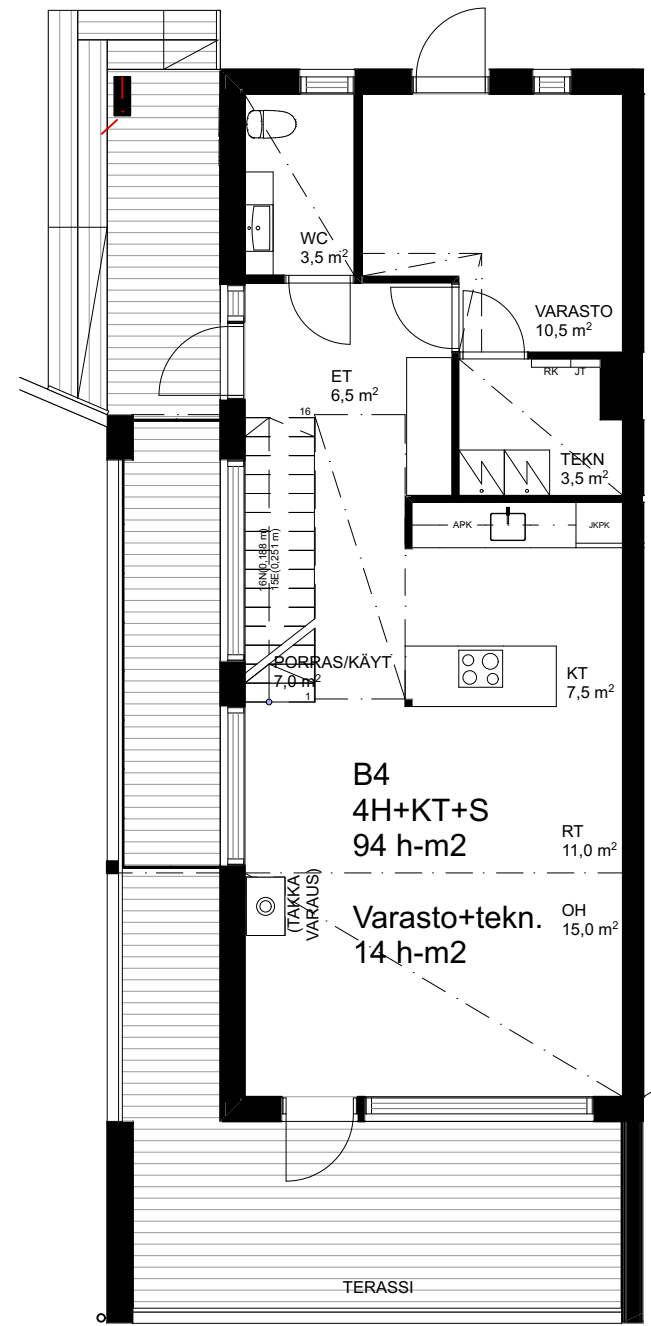
POHJAPIIRROS 1.KRS 1:100
