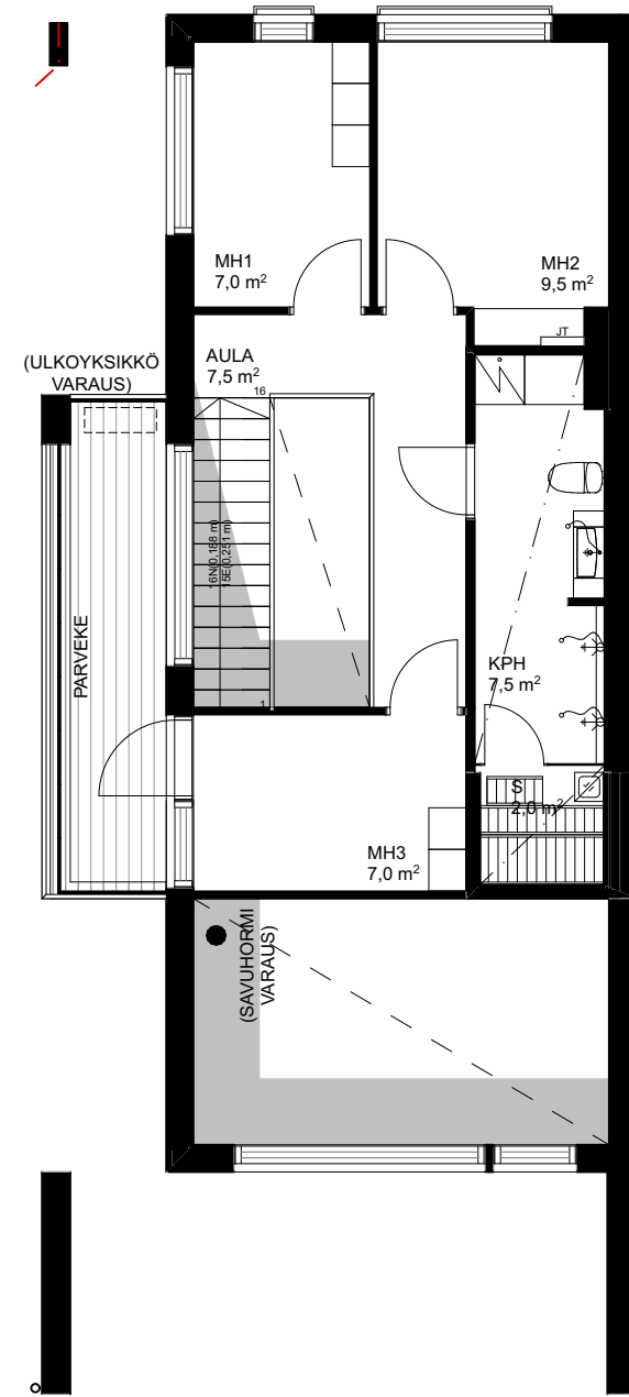
POHJAPIIRROS 2.KRS 1:100
